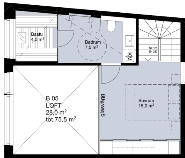
Våning 2
