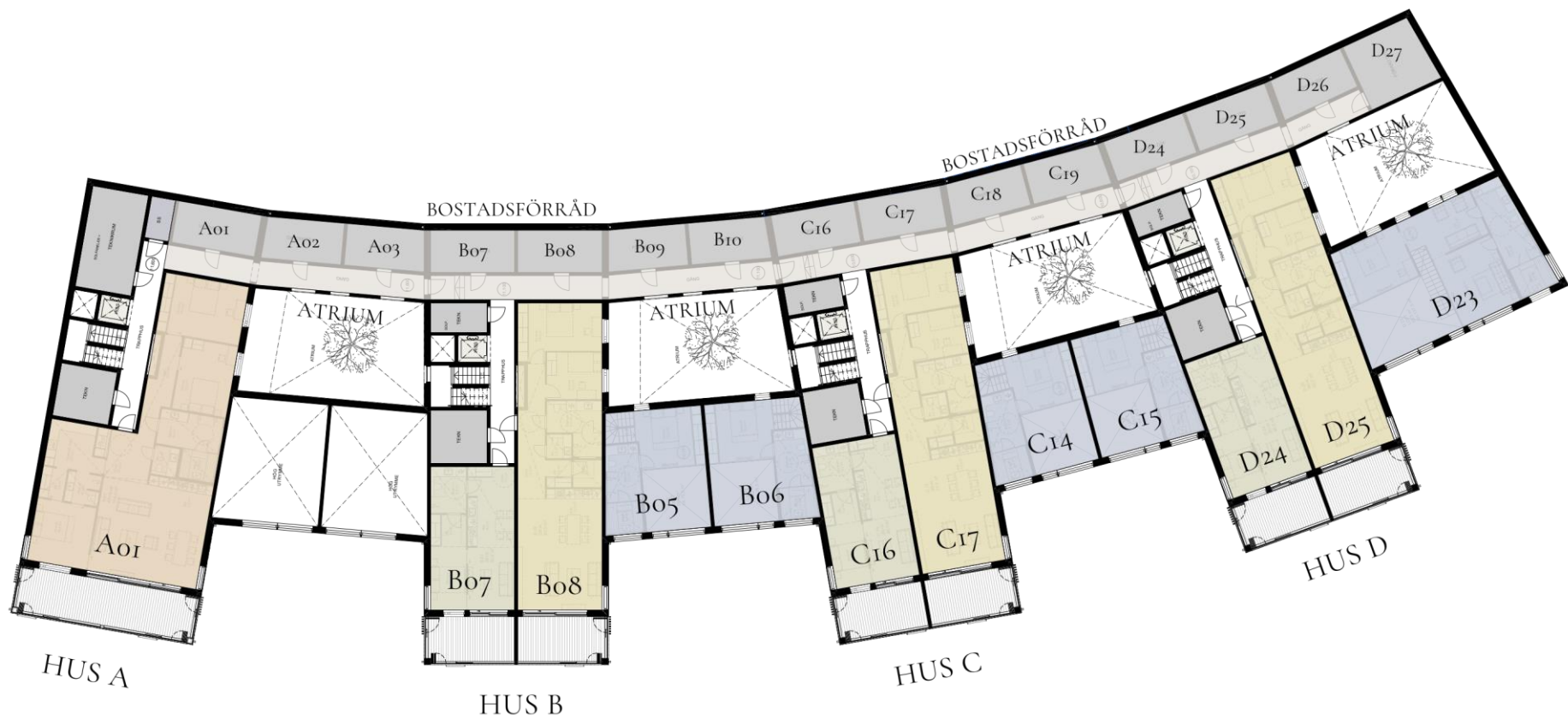
Plan våning 2
